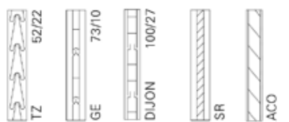
Vue en coupe des persiennes orientables
