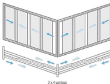
3 rails - Angle rentrant ou sortant
